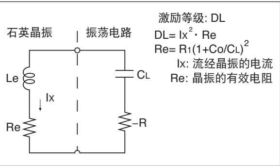
图11 晶振与振荡电路之间的关系
