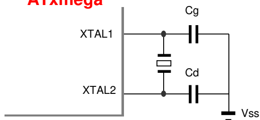
・回路図
