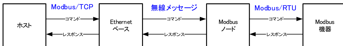
図 7 Modbus/TCP 制御
