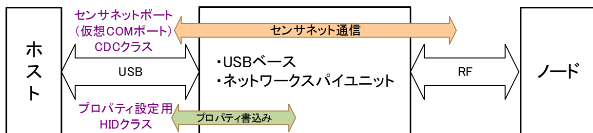
図 5 USB 接続
