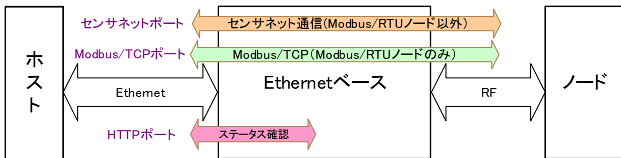
図 2 Ethernet 接続
