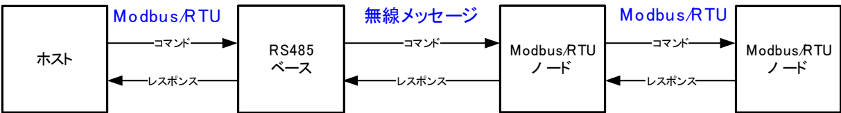
図 9 Modbus/RTU 制御
