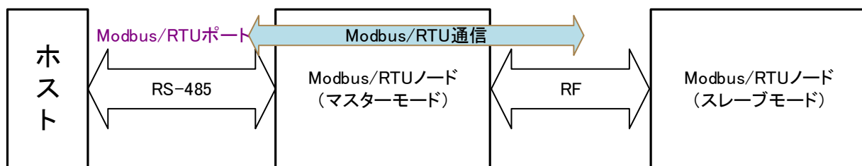
図 4 RS-485 接続
