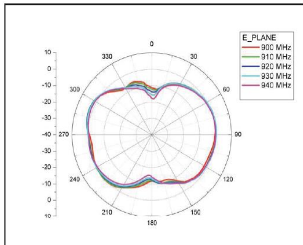
E-plane
