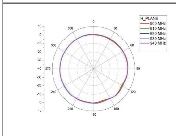
H-plane
