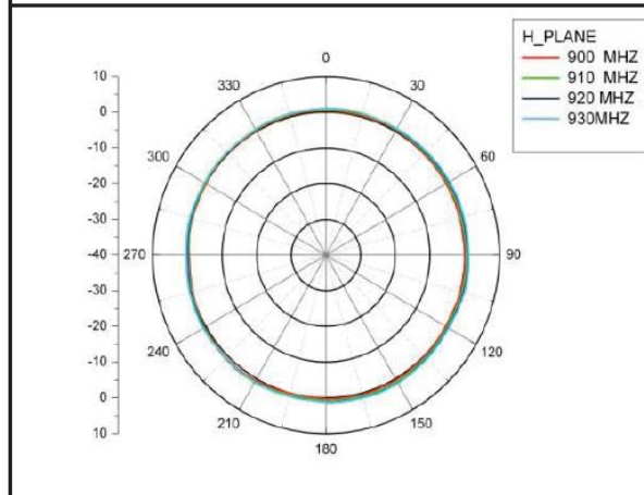
H-plane
