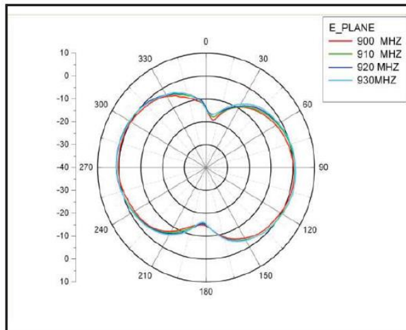
E-plane
