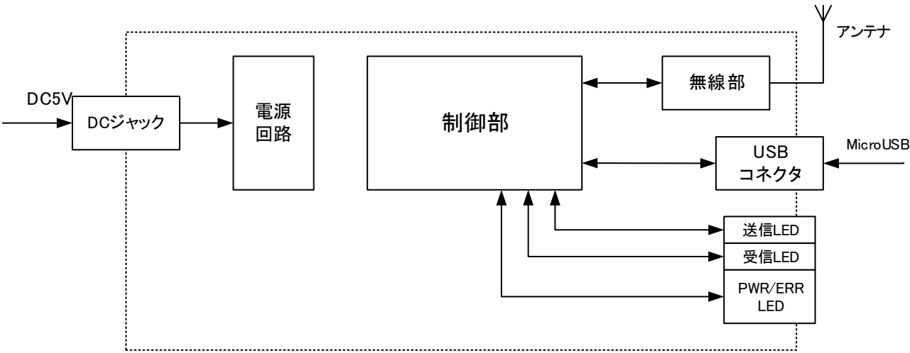
図 3 ブロック図
