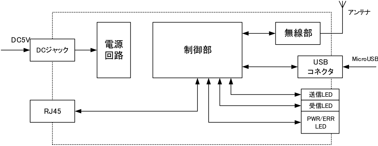
図 3 ブロック図
