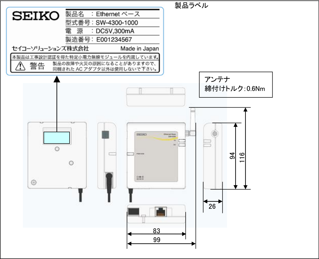
図 4 外形寸法図
