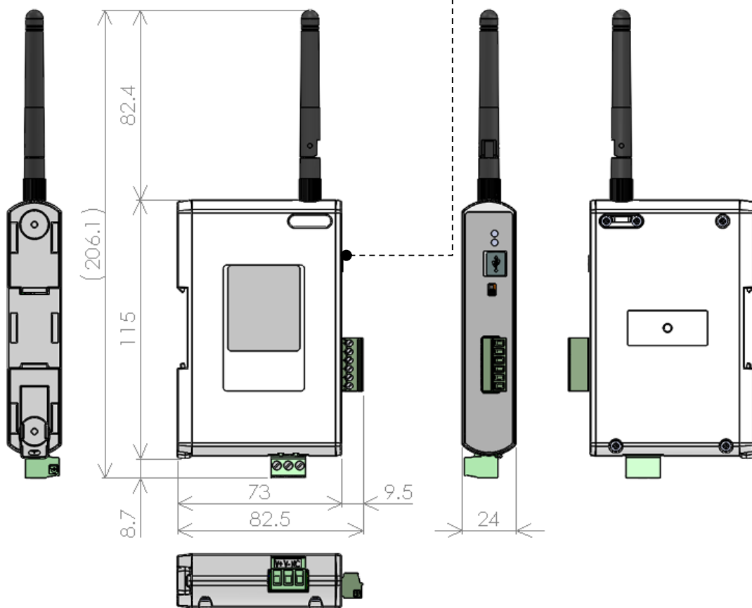
図4 外形寸法図
