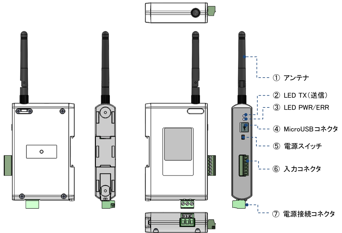
図1 外観と各部の名称
