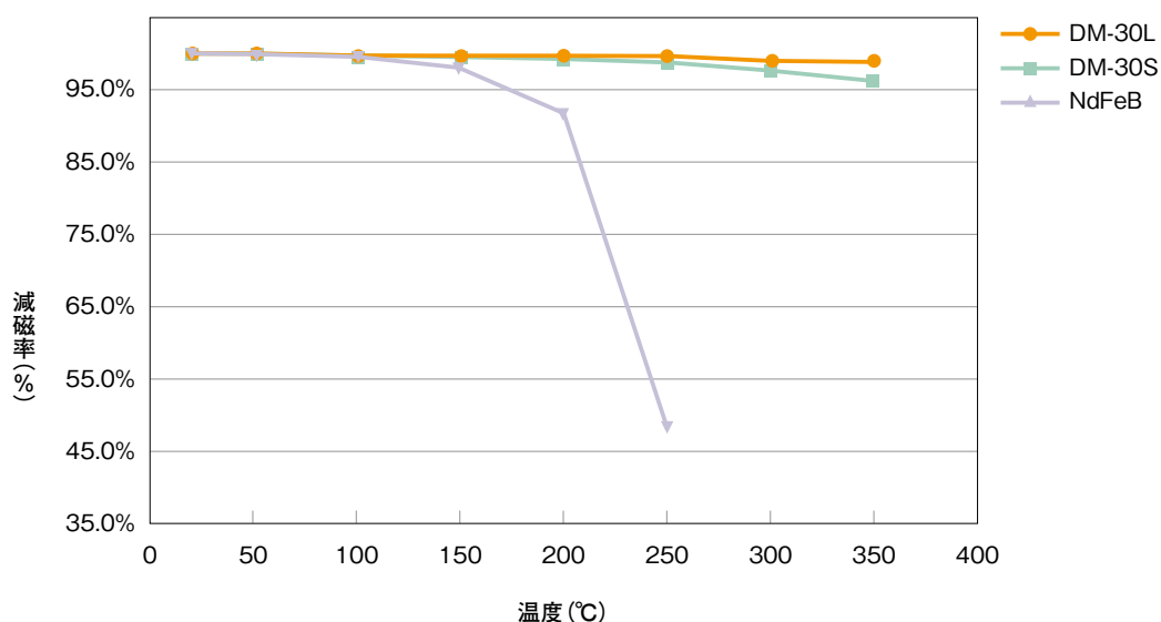
熱減磁率 (FLUX値) の比較
